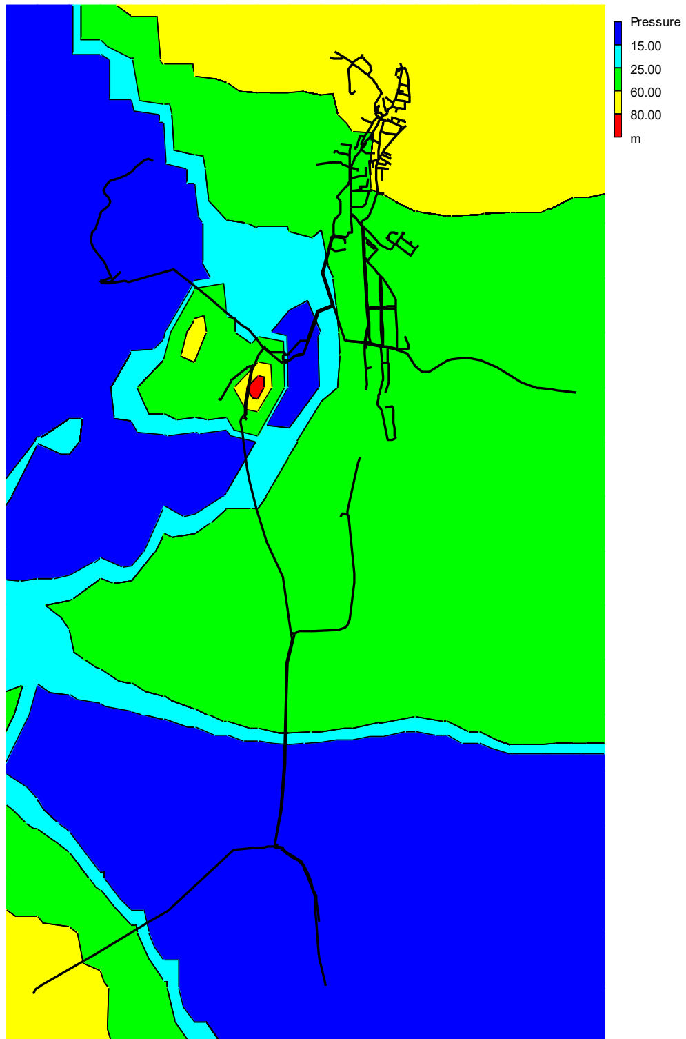
Figura n° 18. Mapa de isólinas de presión bajo la hipótesis de caudal punta
