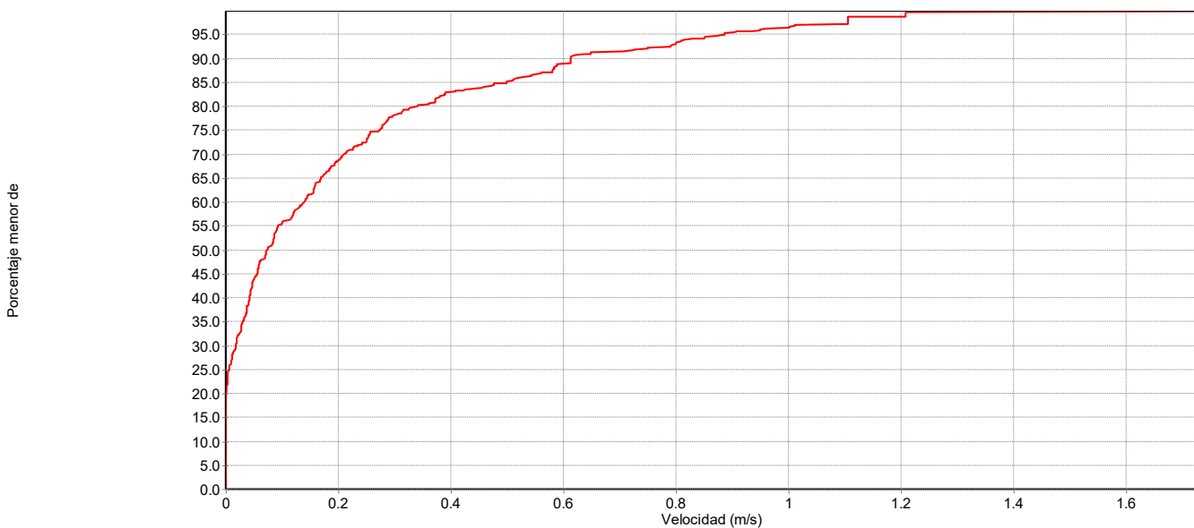
Figura n° 25. Gráfico de velocidades en la red a caudal punta
